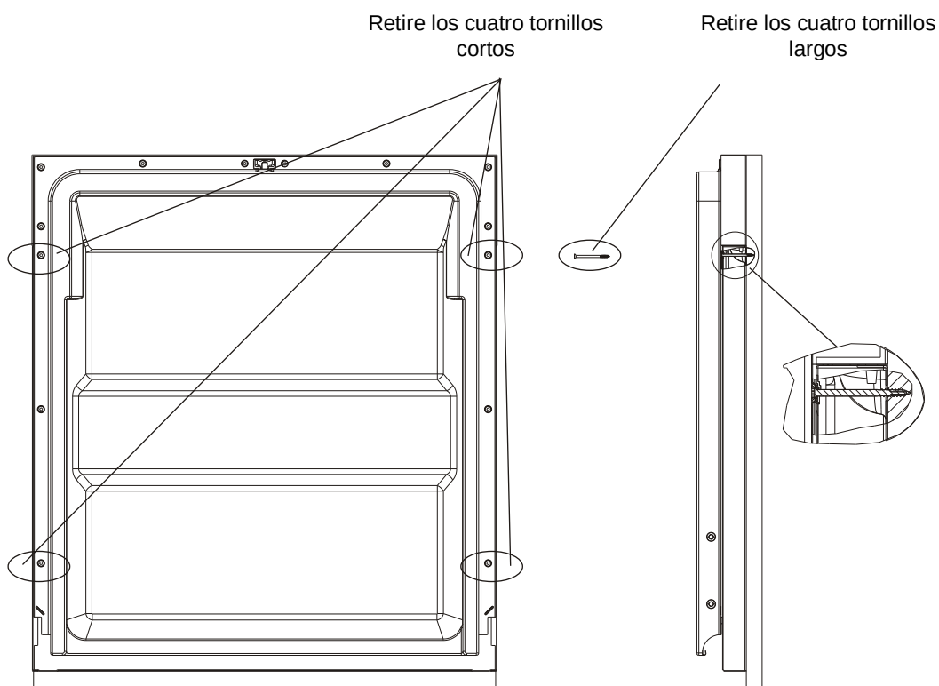
【 Figura 4b 】 Instalación del panel embellecedor de madera
